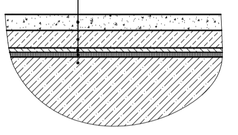
פרט איטום וריצוף
