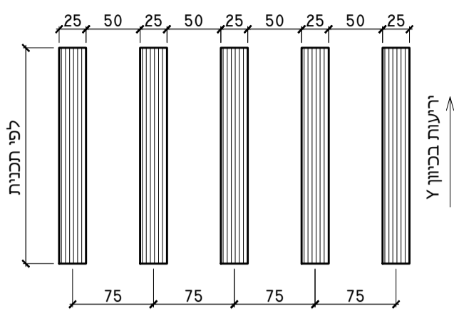
סידור טיפוס של יריעות FRP
