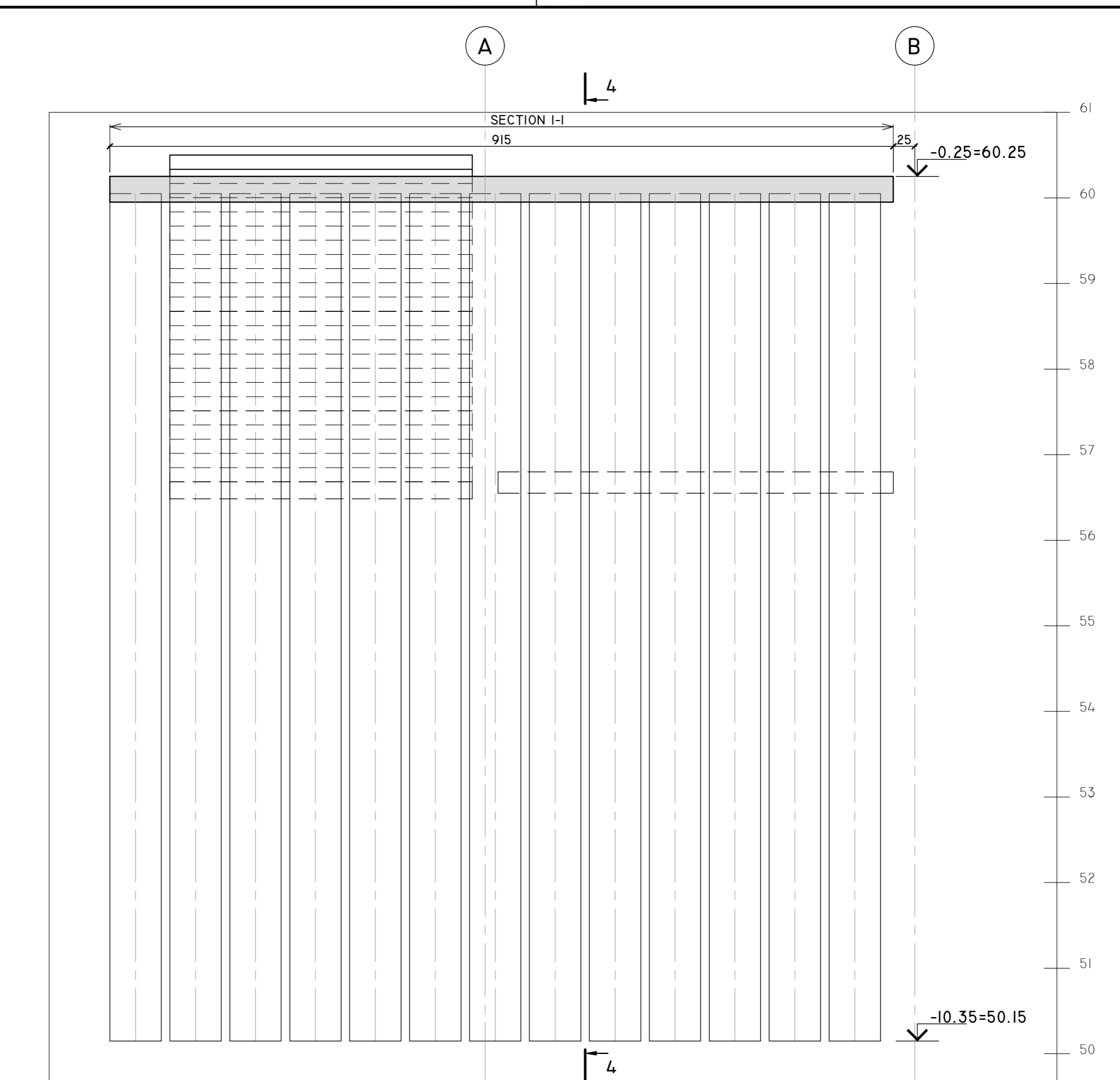
פריסת קיר דיפון צפונית
