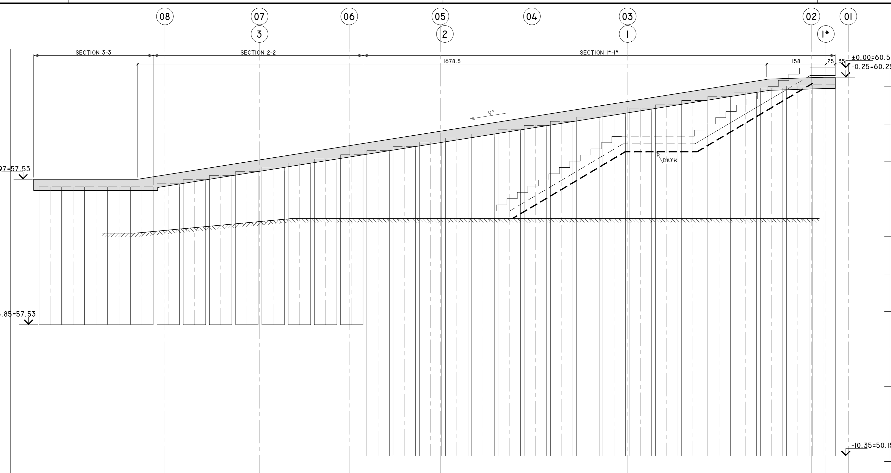
פריסת קיר דיפון מערבית
