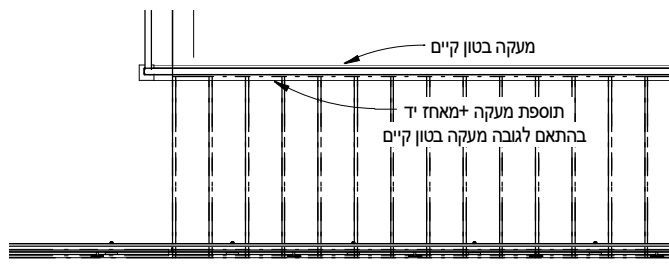
1 תוכנית
