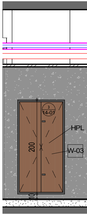
חזית
