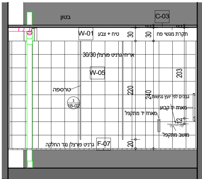
חזית 4 קנ"מ: 1 : 50 71-18
