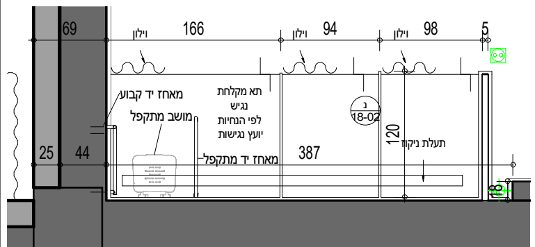
תכנית 3 קנ"מ: 1 : 50 71-18
