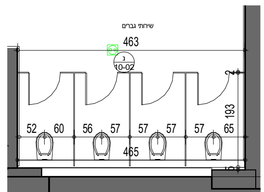
תכנית 3
