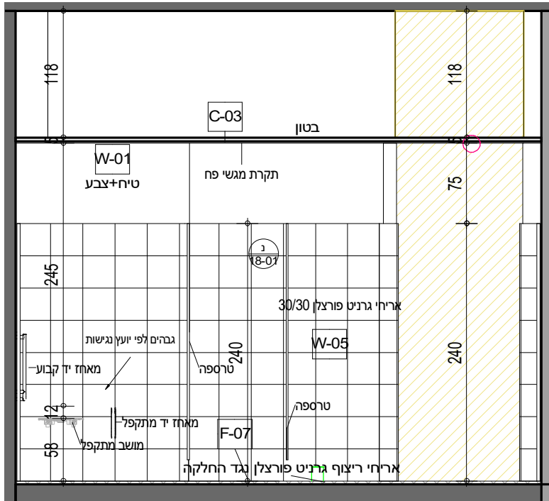
חזית 1 קנ"מ: 1 : 50 71-18
