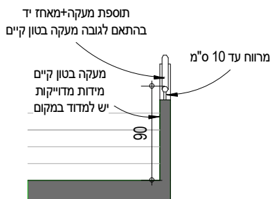
2 חתך
