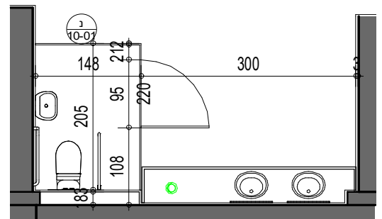
תכנית 1
