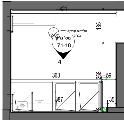
תכנית
