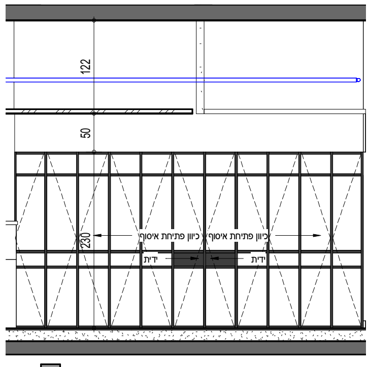
2 חזית
