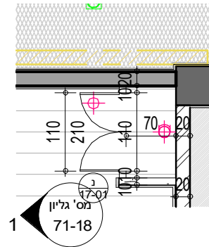
תכנית
