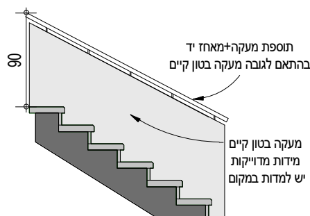
3 חזית
