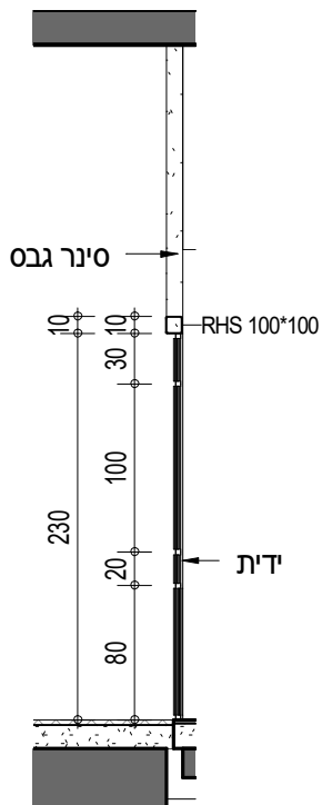
3 חתך
