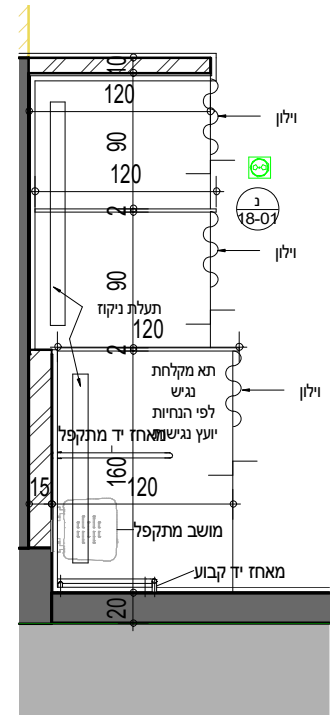
תכנית 2 קנ"מ: 1 : 50 71-18
