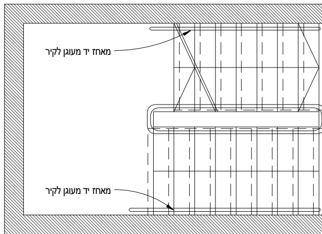
תוכנית
