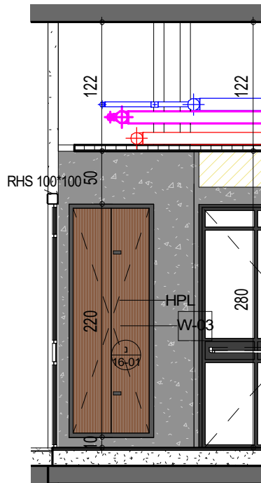
חזית
