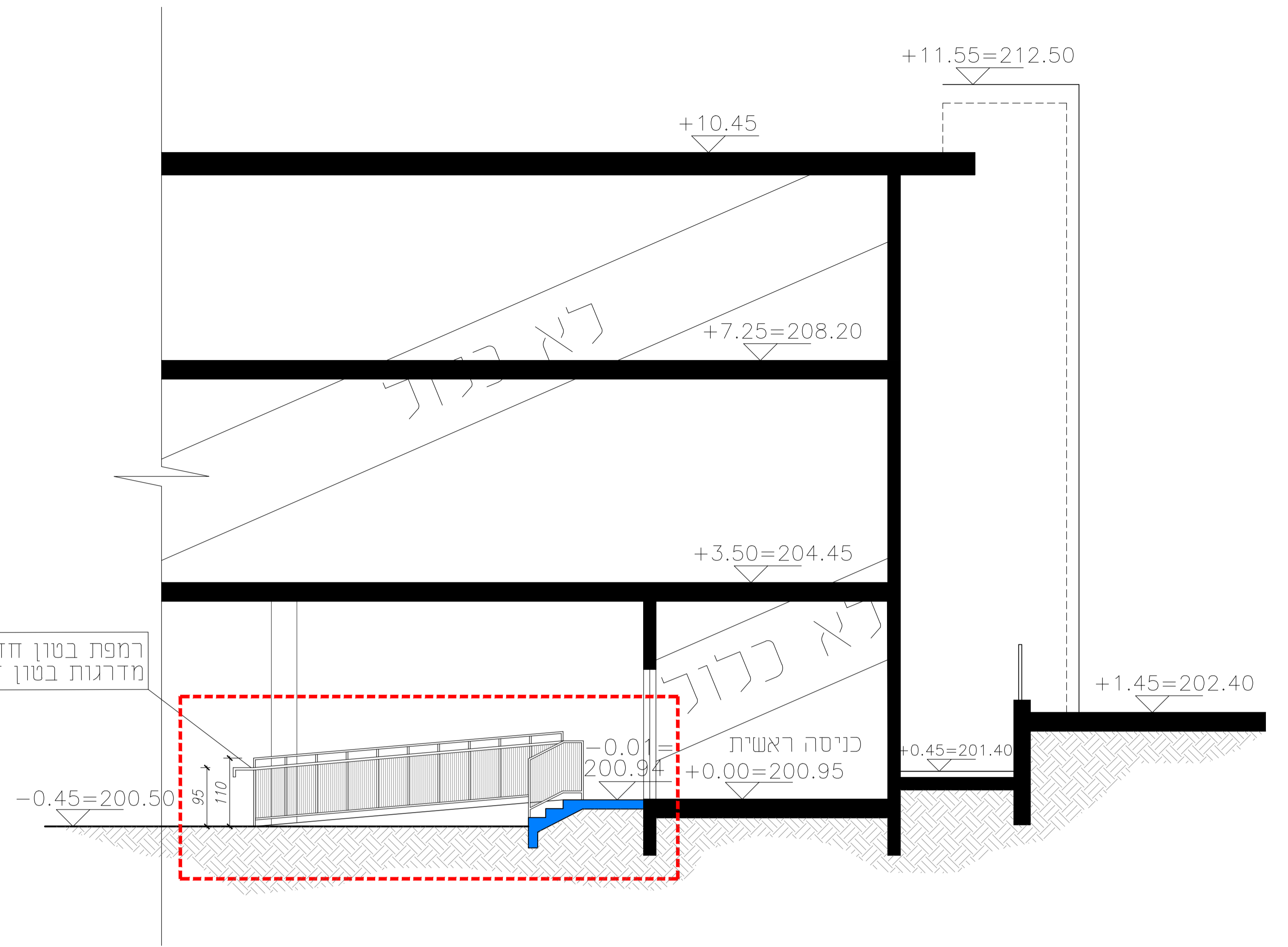
חתך 3-3
